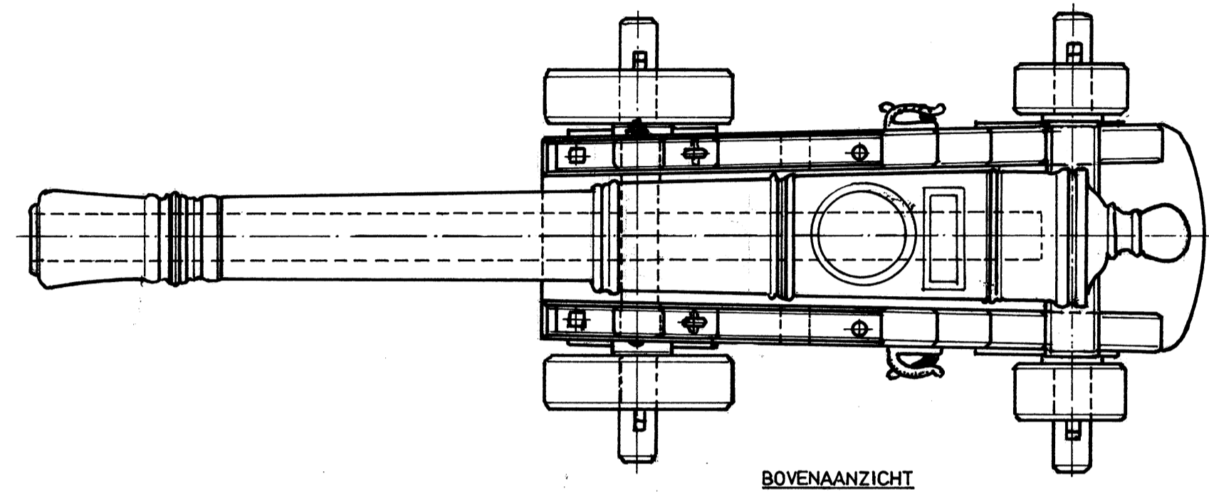
BOVENAANZICHT
