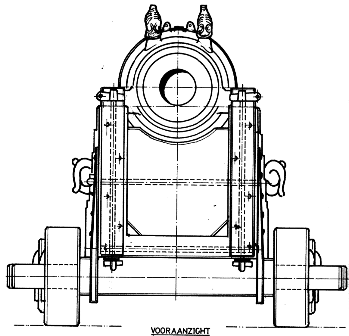
VOORAANZICHT
