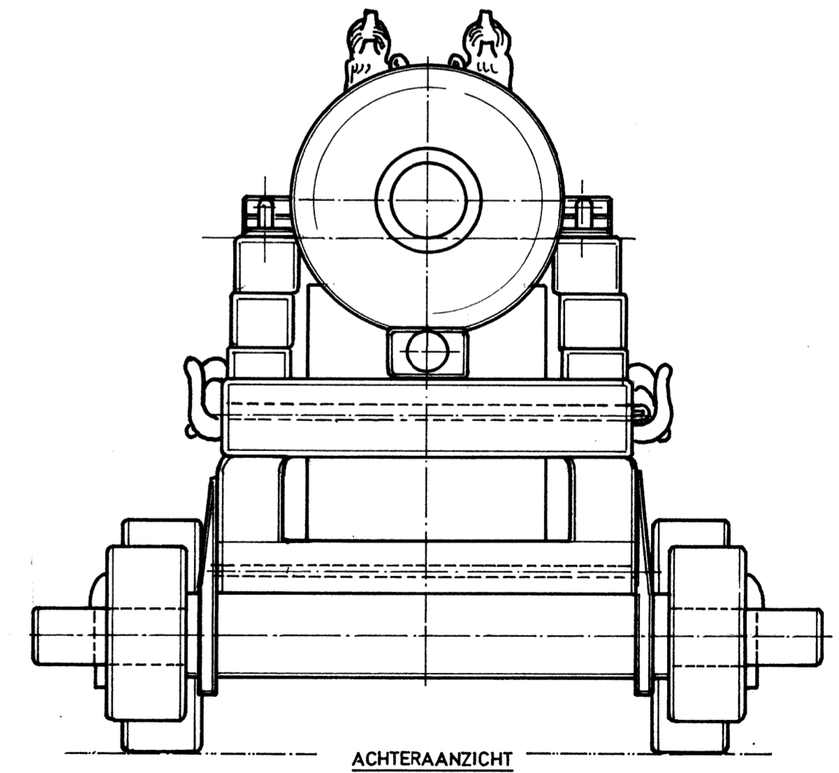
ACHTERAANZICHT
