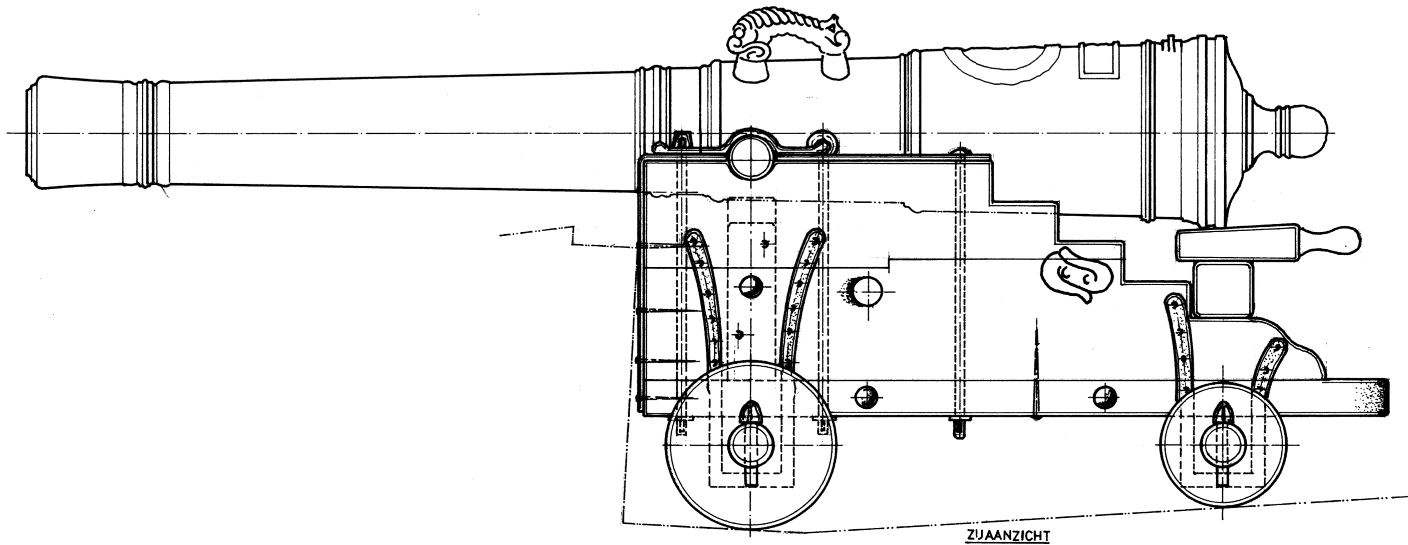
ZIJAAANZICHT
